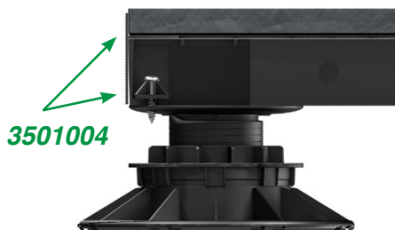
Fixácia mriežky (3501000) na podstavec
