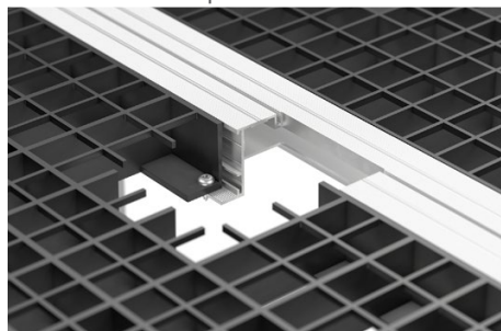
Fixácia mriežky (3501000), do hliníkového rámu
