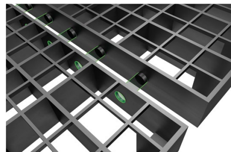
Detail bočných zámkov medzi mriežkami
