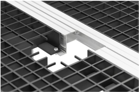
Fixation de la prédalle (3501000), encastrée dans le cadre en aluminium
