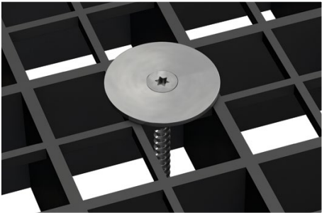
Clip en aluminium (3501005), fixation intermédiaire des prédalles (3501000)
