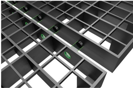
Détails de la fixation latérale entre les prédalles
